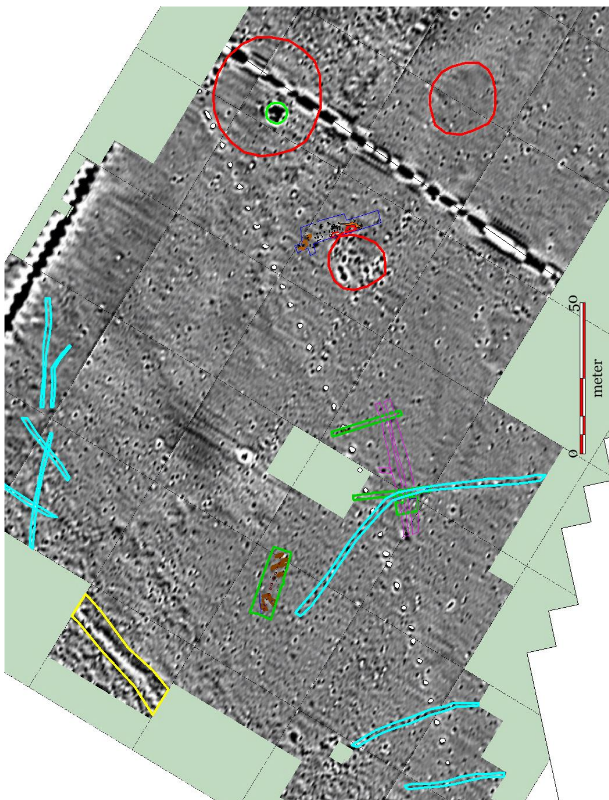
Figur 26. Magnetometerkartering med tolkningar och schakt. Röda cirkelar gravar, Ljusgrön ring plundringsgrop, Ljusblå diken, gula streck vägdike, gröna streck schakten från 2016, blåa streck schaktet från 2017, lila streck utbredning av väglikande struktur, de vita punkterna visar vattenledningens utsträckning. Genom området löper två elledningar som ger kraftiga svartvita markeringar, en av dessa går genom den stora graven Raä 104:1.
