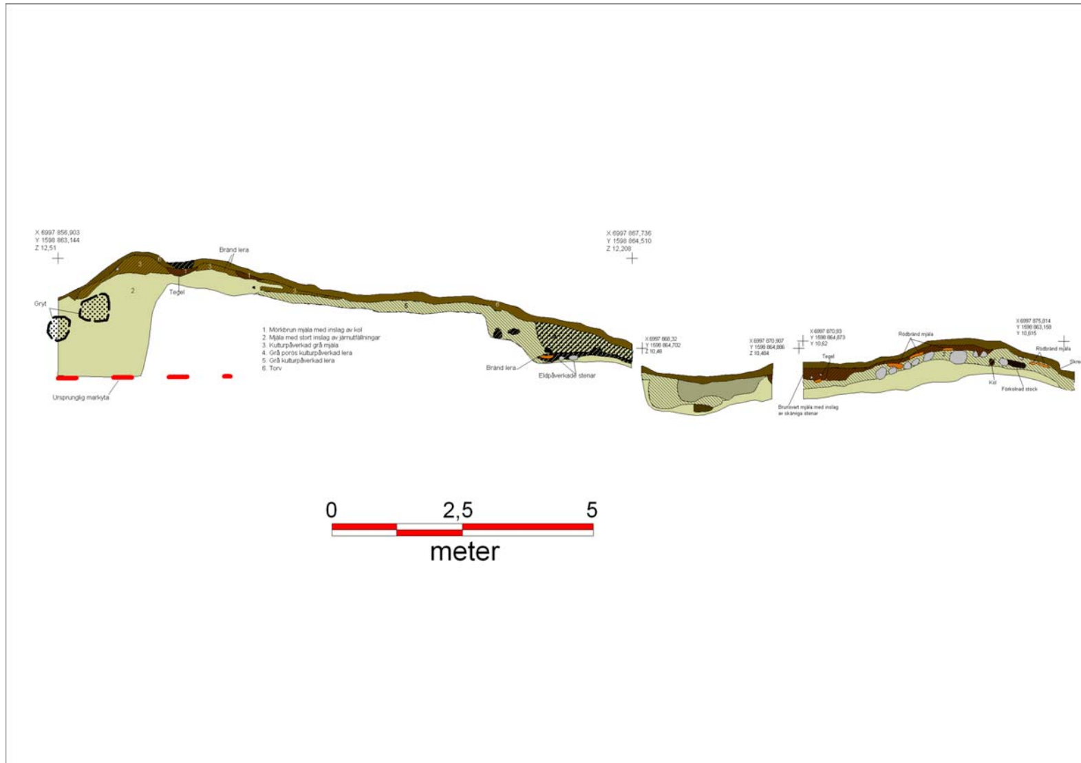
Hela långprofilen.
