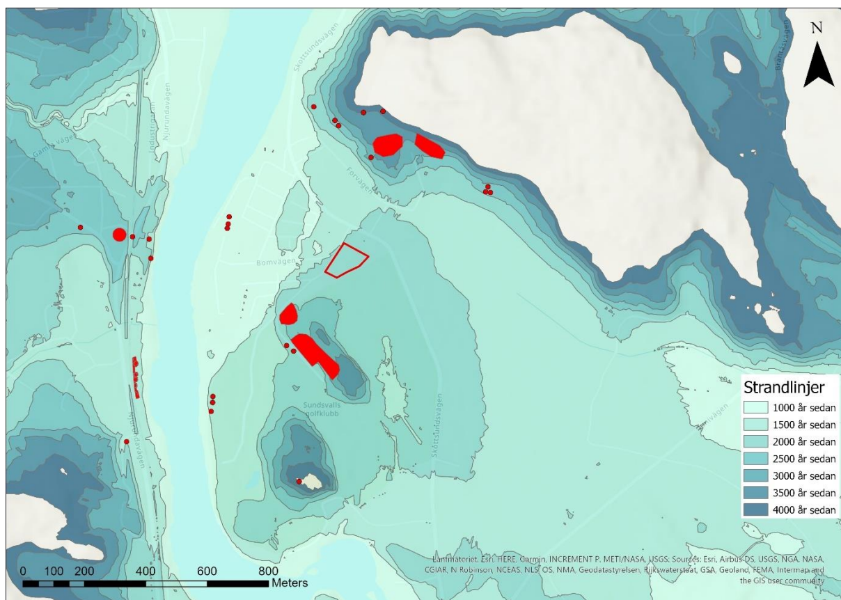
Figur 2. Strandlinjer för olika perioder kring utredningsområdet. Nordväst om utredningsområdet är området starkt påverkat av bebyggelse. © ESRI
