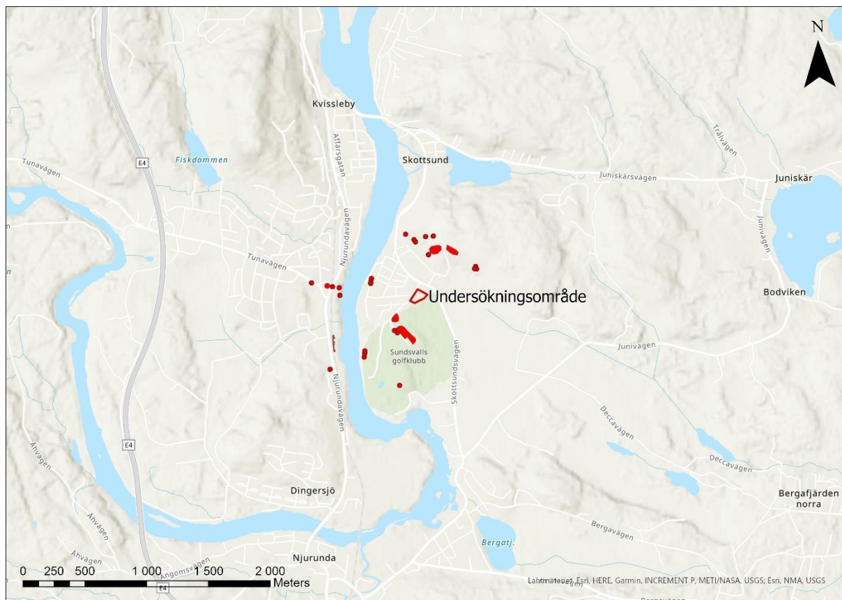
Figur 1. Utredningsområdets geografiska läge. © ESRI
