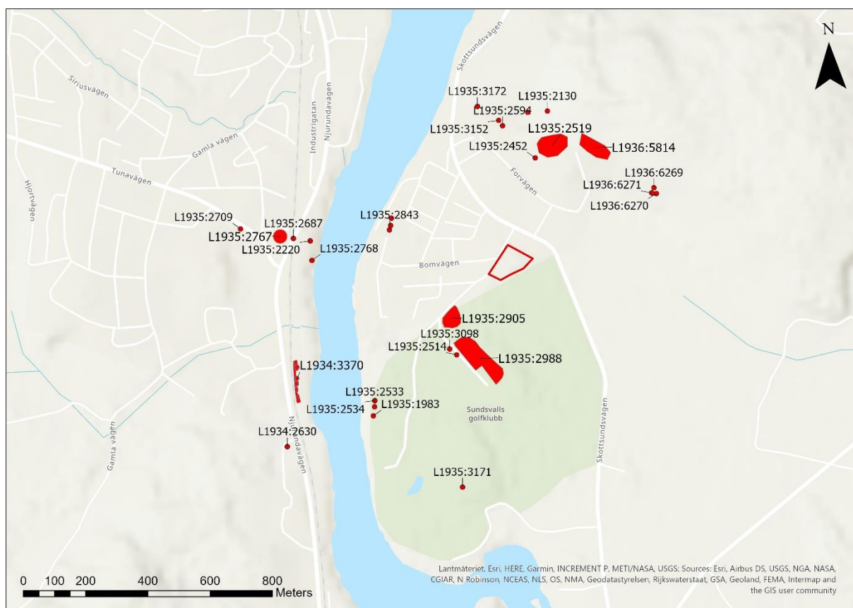
Figur 3. Fornlämningar kring utredningsområdet. © ESRI
